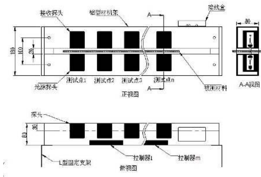
图 3.1 LS152 测控主机结构示意图
