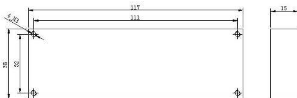
图 8.5 控制器安装尺寸图
