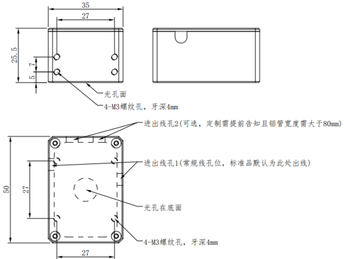
图 8.3 接收探头安装尺寸图
