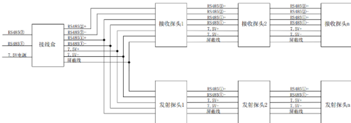
图 8.1 测控主机内部连接示意图
