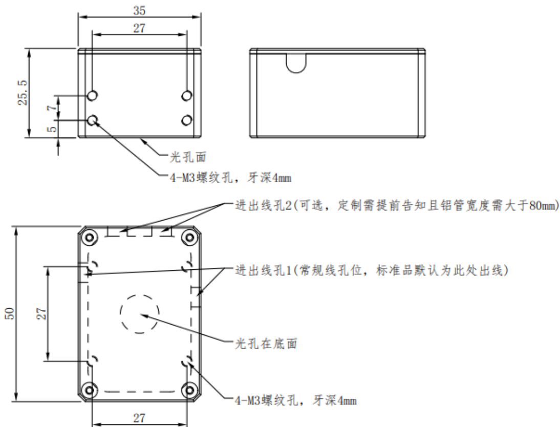
图 8.3 接收探头安装尺寸图
