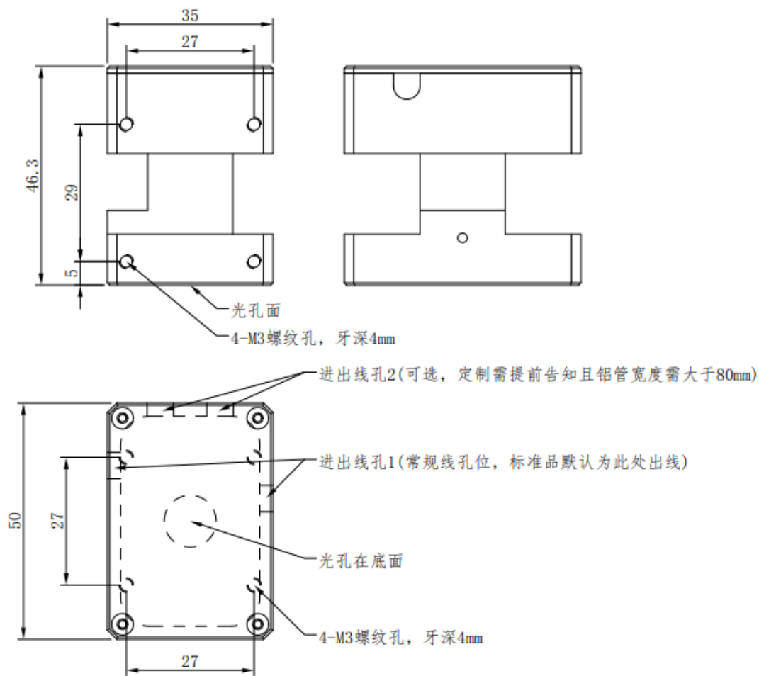
图 8.2 光源探头安装尺寸图
